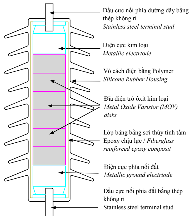
Mặt cắt bên trong của chống sét Cutaway View of Typical Unit
