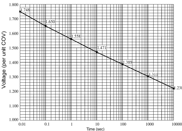
Khả năng chịu quá áp tạm thời - TOV Capability
